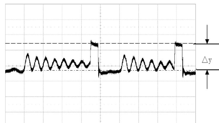
图 18 共模噪声波形示意图（三）
